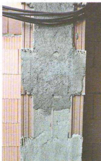
Monolithische Bauweise: Kompakte Wand mit speziellen Mauerziegeln gebaut. Der Hohlraum der Ziegeln ist gefüllt mit wärmedämmendem Material.
